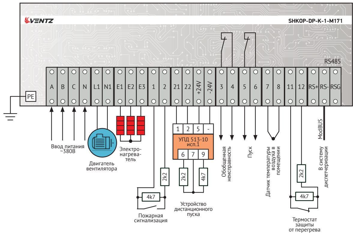
Схема подключения
