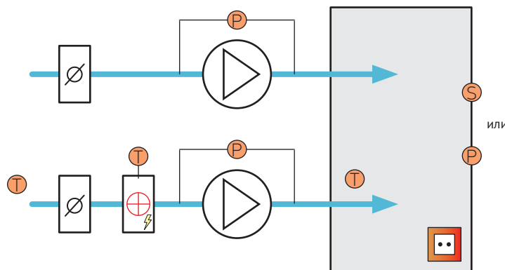
Структурная схема установки
