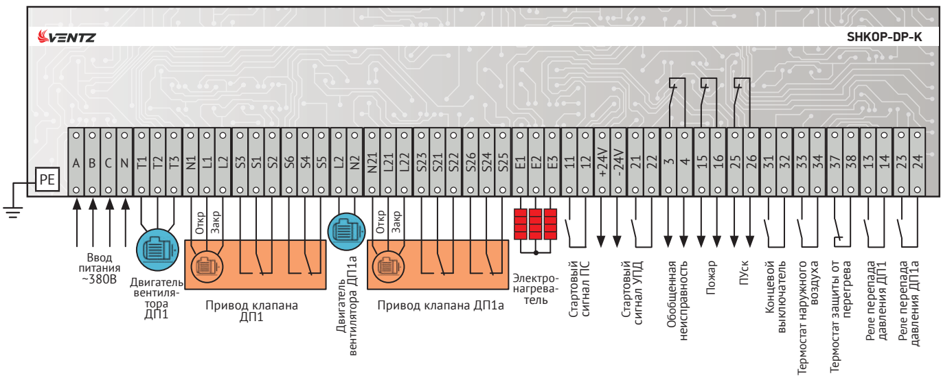
Схема подключения
